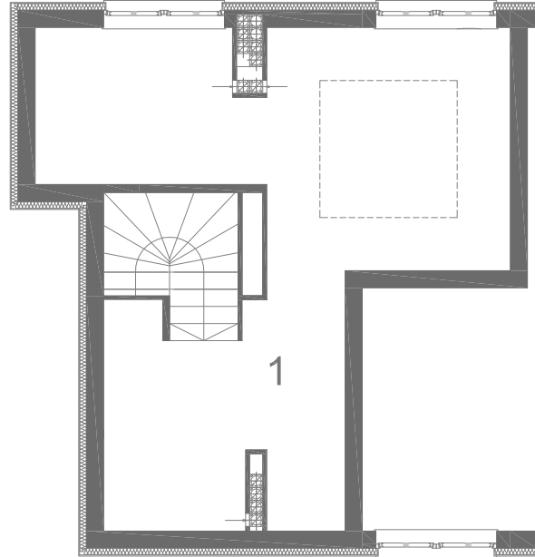
POZIOM II
